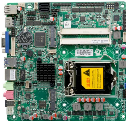
ITX-D81_D6L VER:1.0 主板正面图
