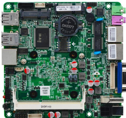
STX-N39_19 VER:1.2A 主板正面图
